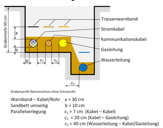
Bild 4 Gemeinsame Hausanschlussstrasse auf dem Privatgrundstück
