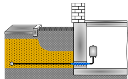
Bild 5 Gebäudeeinführungen Beispiele für Hauseinführungsvarianten (Gas- und wasserdichte Ausführung nach DIN 18322, DIN 18195 und DIN 18012)
